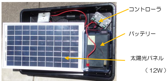
【図2】 自宅で稼働中のミニ太陽光発電システム
